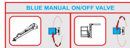
Figure 19 vanne bleue pour échange d'alimentation stabilisateurs/partie aérienne.
