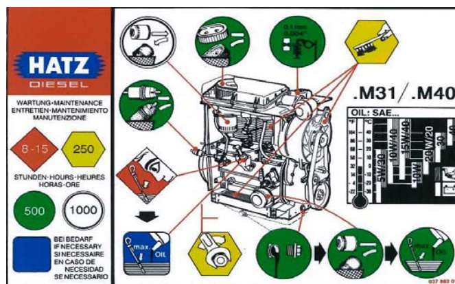
Autocollant des consignes d'entretien pour le moteur diesel
